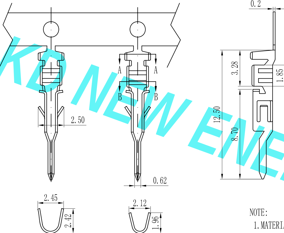
A-A SEC
