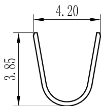
A-A SEC
