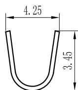
A-A SEC
