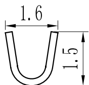
A-A SEC
