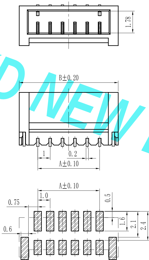
P.C.B LAYOUT
