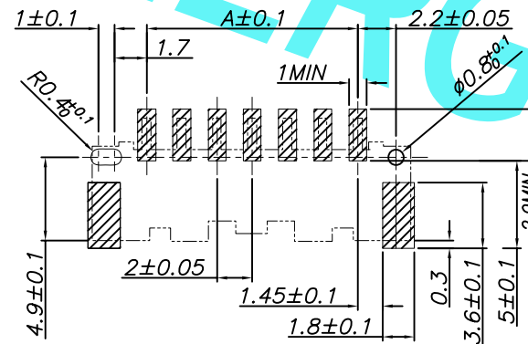
P.C.B. LAYOUT
