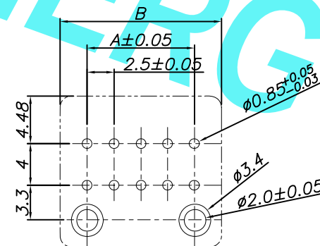
P.C.B. LAYOUT
