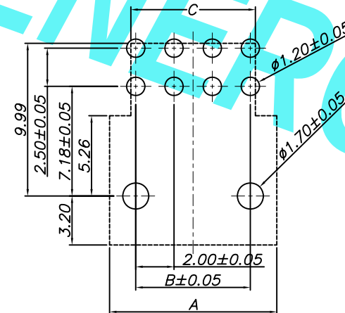
P.C.B. LAYOUT
