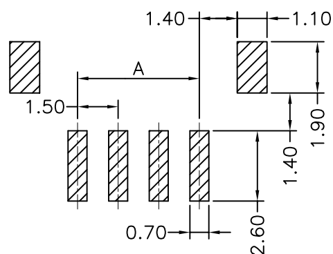
P.C.B. LAYOUT
