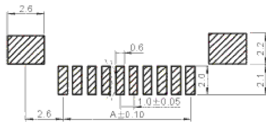
印制线路板 P.C.B. Layout
