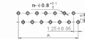
反针 PCB 寸法 Versa needle PCB LAYOUT
