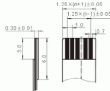
适用扁平电缆 Proper cable
