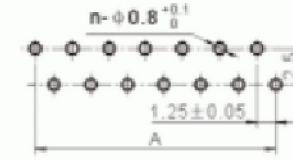
反针 PCB 寸法 Versa needle PCB LAYOUT
