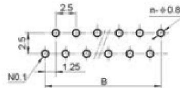
印制线路板 P.C.B Layout
