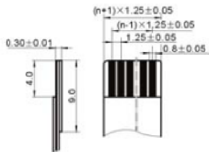
适用扁平电缆 Proper cable
