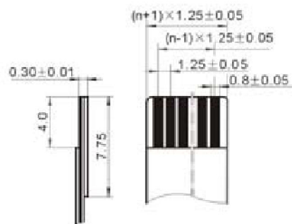
适用扁平电缆 Proper cable
