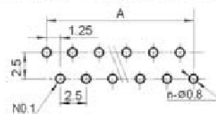
反针 PCB 寸法 Versa needle PCB LAYOUT
